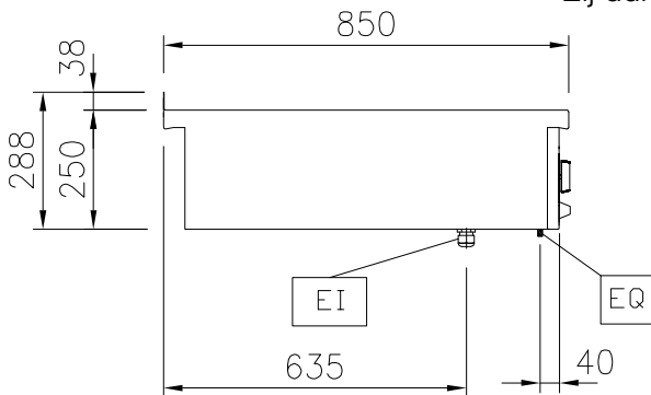
Zij aanzicht
